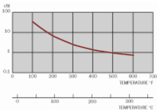
В'язкість
