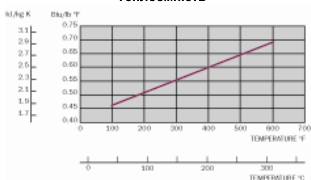
Теплосмієність
